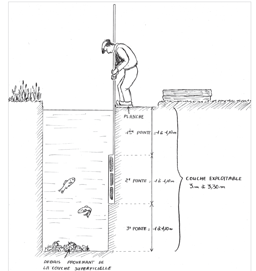
doc. 4 L'extraction de la tourbe au louchet. Dessin Jean Maclin
