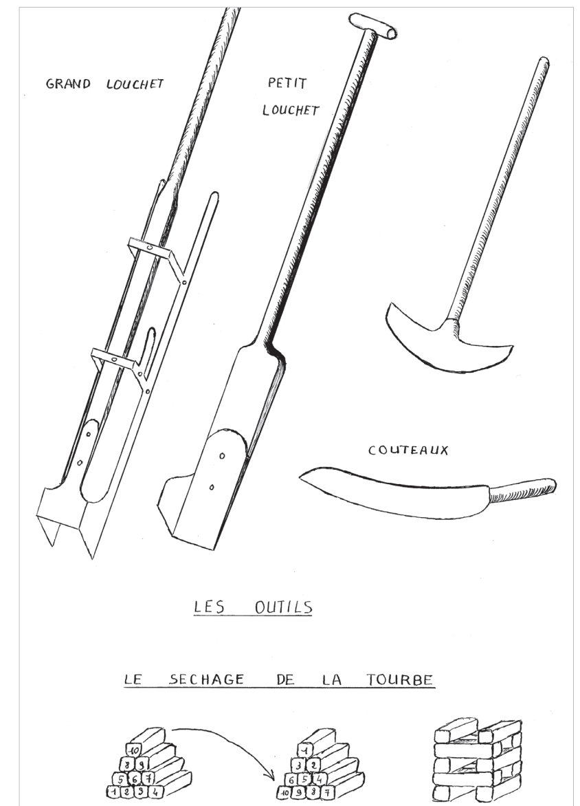
doc. 6 Les outils de la tourbe et le séchage de la tourbe. Dessin Jean Maclin
