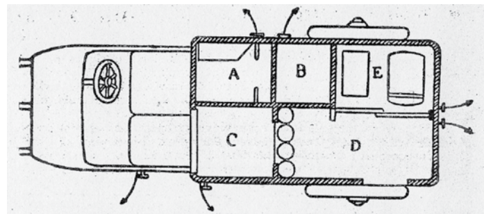
doc.1 Coupe d'une voiture automobile chirurgicale, Le Pays de France , 1 er mars 1917.
